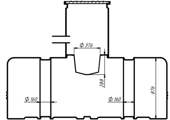
CROSS-SECTION A:A SCALE 1:12
